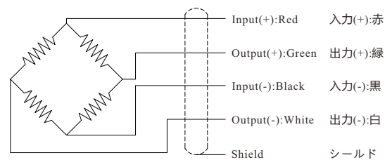
Wiring Diagram/配線図
