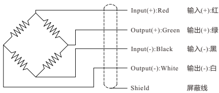
Wiring Diagram/接线图
