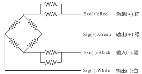
Wiring Diagram/接线图
