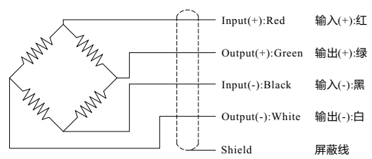
Wiring Diagram/接线图
