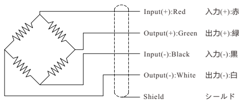
Wiring Diagram/配線図
